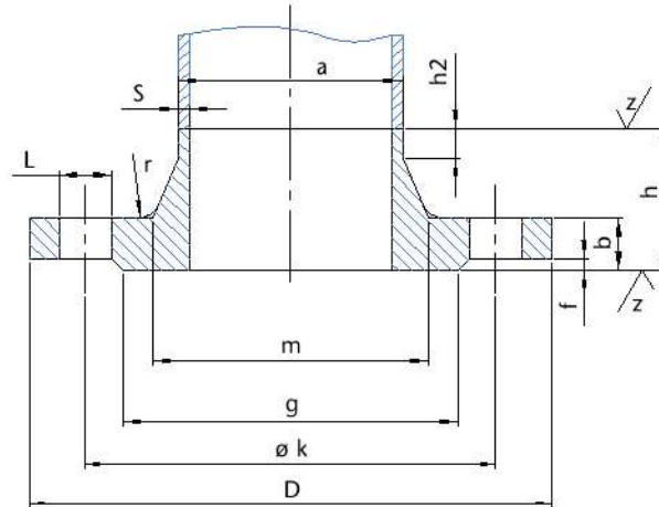
EN 1092-1 tipo 11 PN25/40
